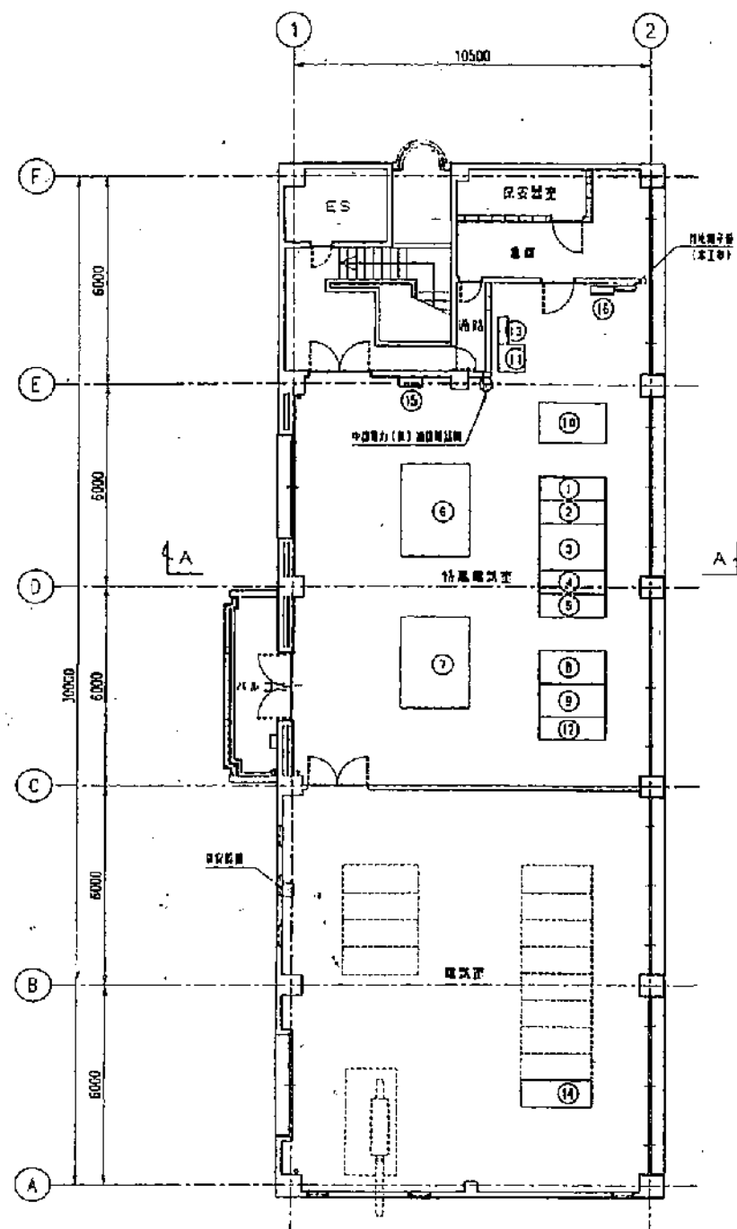
機器配置図 S=1/100
