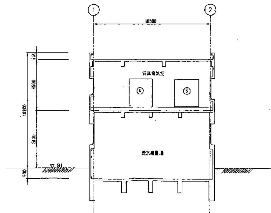
A - A 断面図 S=1/100
