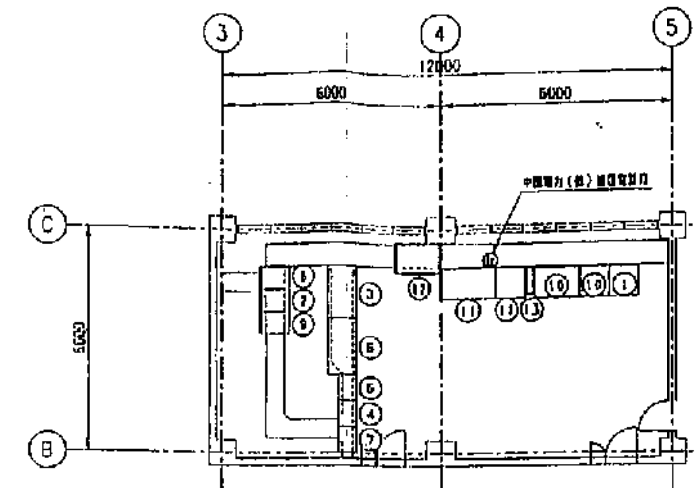
中央監視室(管理棟)平面図 S=1/100
