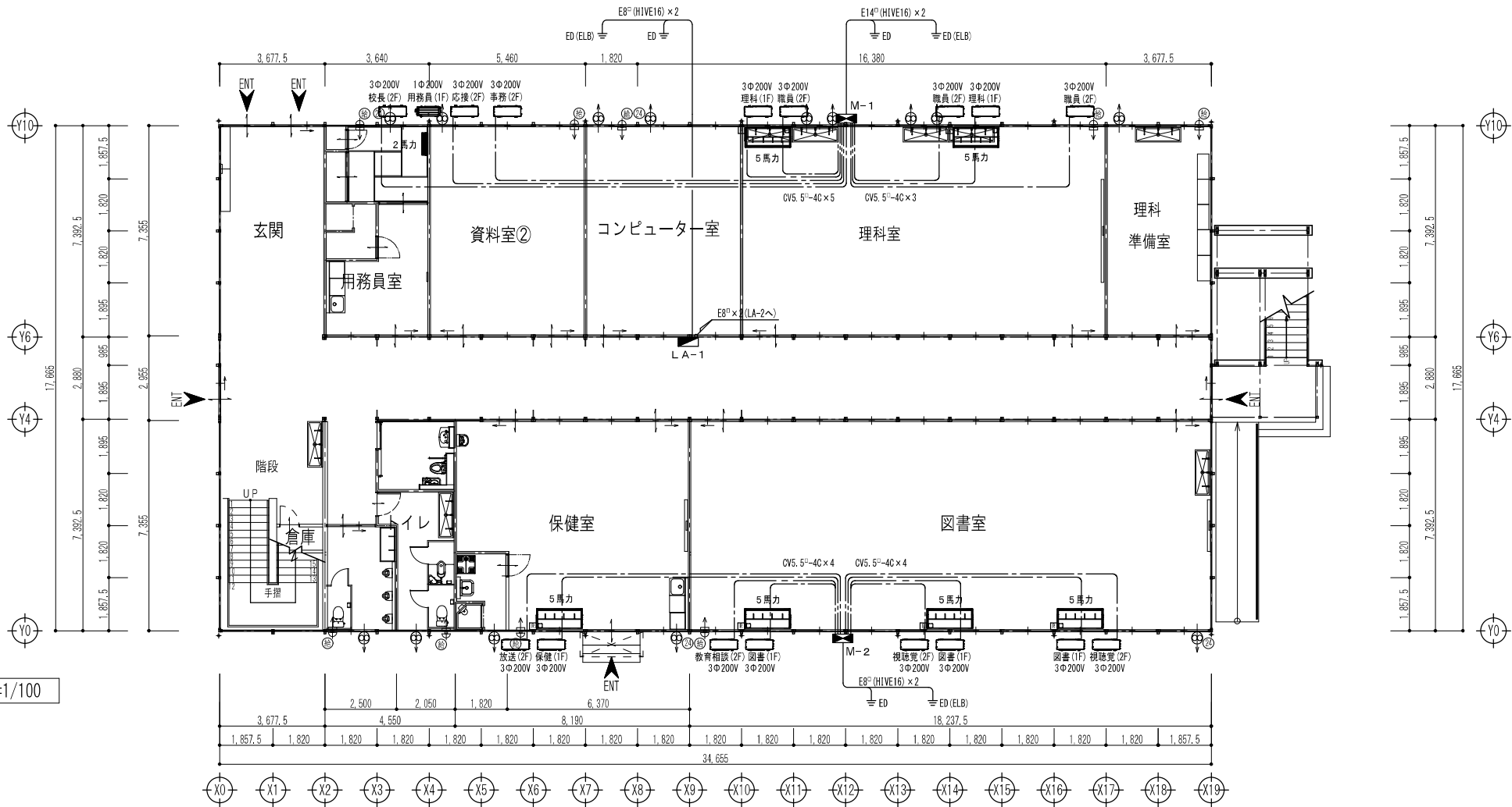
動力盤 (M-1)
