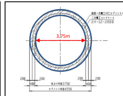
図-1 完成した雨水管の断面図
