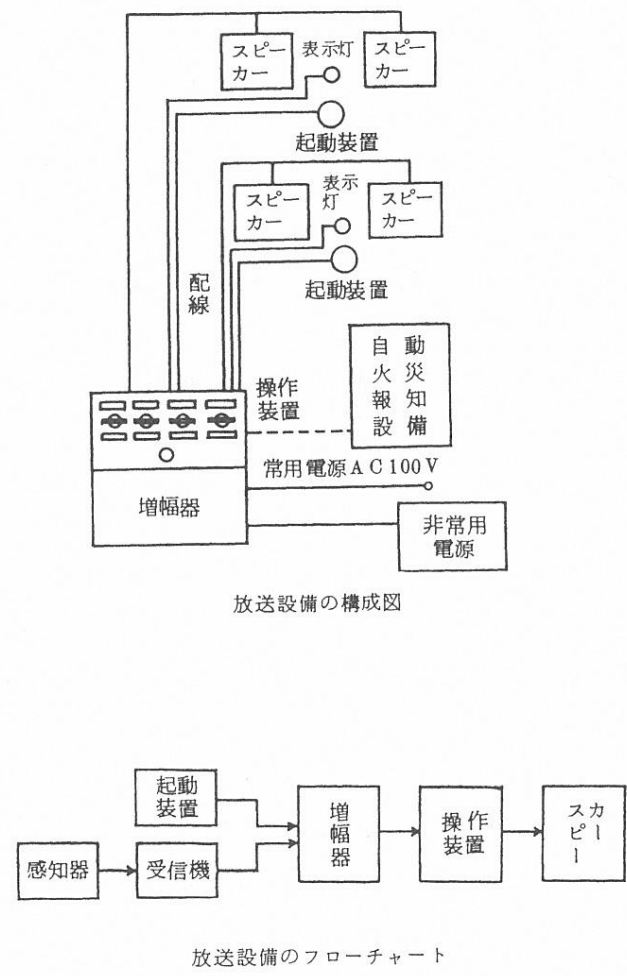
図14-4 非常放送設備の概要
