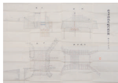
弥五平脇改築樋門設計図
